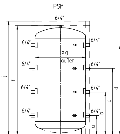
PSM - Pufferspeicher mit 6/4" - Anschlussmuffen 500 - 5000l
